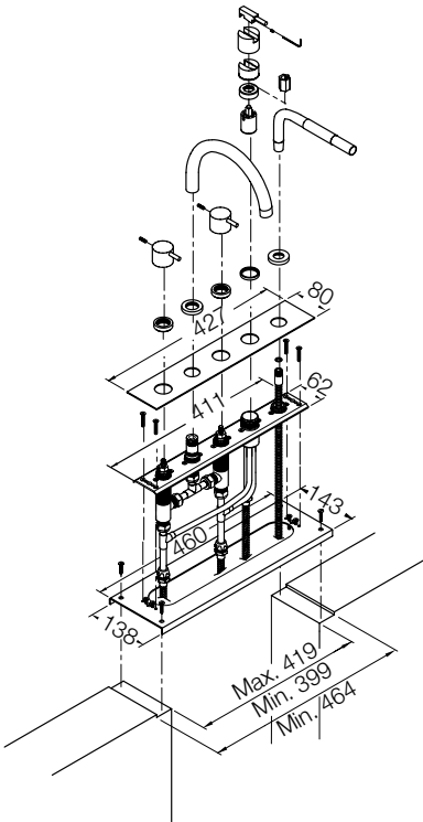
Même modèle que BK sans structure porteuse et sans boîte de sécurité (type BKA).
