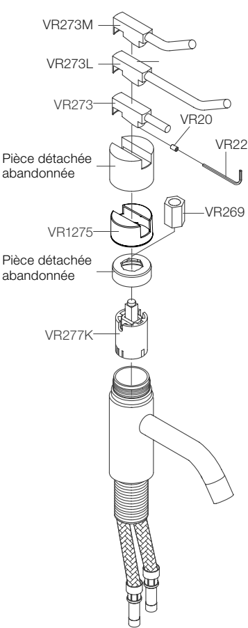
Bonde et poignée fabrication antérieure à 2011
