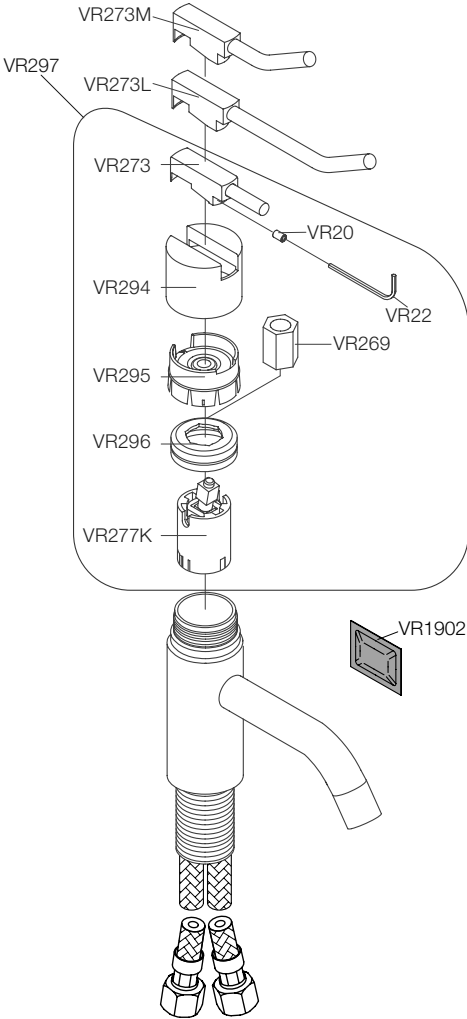
Bonde et poignée fabrication ultérieure à 2011
