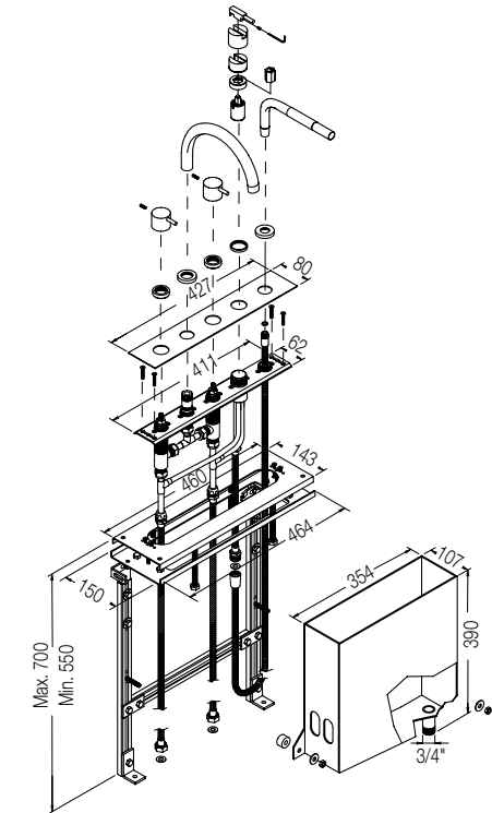
Combinaison complète système extractible avec boîte de sécurité (type BK).
