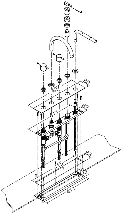
Même modèle que BK avec une installation directe sur le bord de la baignoire (type BKB).
