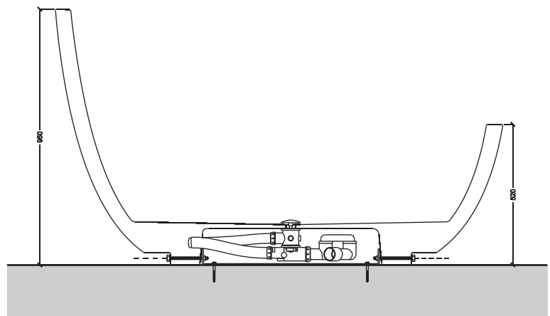
Sezione A-A'
